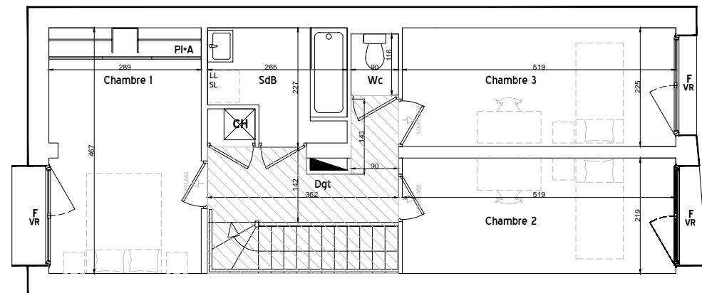
PLAN ETAGE
